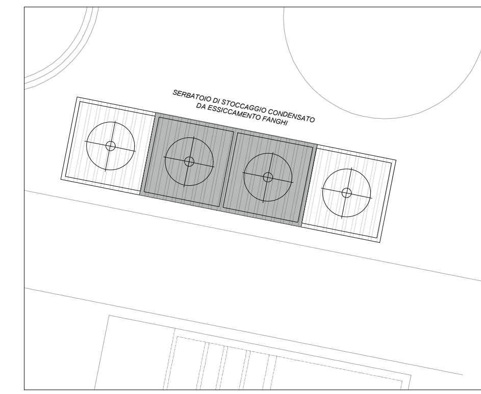
ESTRATTO PLANIMETRICO (D-10-230 - Planimetria generale impiantistica)
